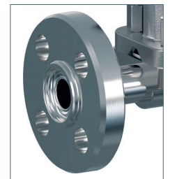
N = Flange with groove DIN 11864-2 Form A
