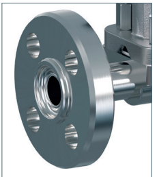
N = Bride avec rainure DIN 11864-2 Forme A
